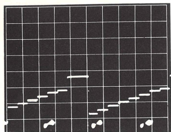
50V div 10µs div
