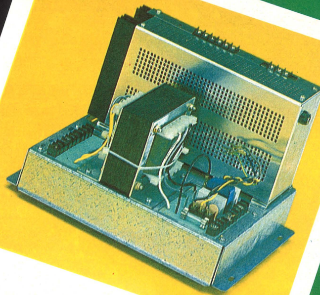
ALIMENTATORE UNIVERSALE PSB 100A - permette l'alimentazione del monitor-colore, delle lampade della gettoniera, dei neon, e di supportare l'alimentatore Switch US 100 UNIVERSAL POWER UNIT PSB 100A - supplies the colour monitor, coin mechanism lamps, neons and feeds the Switch-Mode Power Supply US 100.
