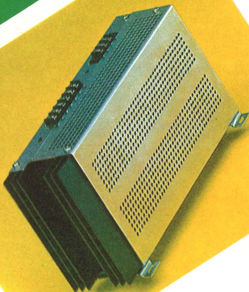
US 100 Alimentatore basse tensioni per Piastre della Logica Low voltage Power Unit for Logic Board AC 117/240+5V.7A/-5V.1A/+12V.1.5A/-12V.0.5A
