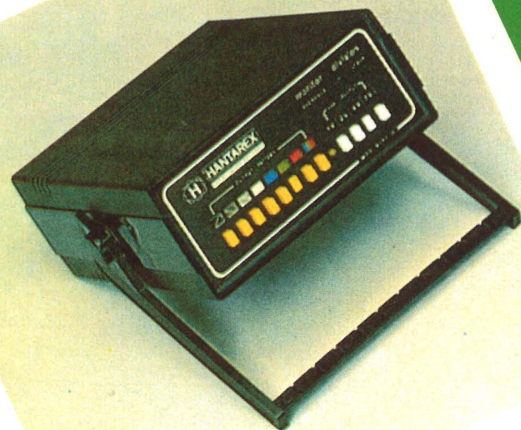
K 190 G Generatore di segnali RGB per il controllo e la messa a punto di monitors a colori RGB signal generator for testing and setting-up colour monitors
