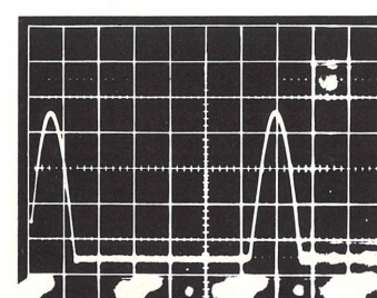
200 Vpp div 10µs div
